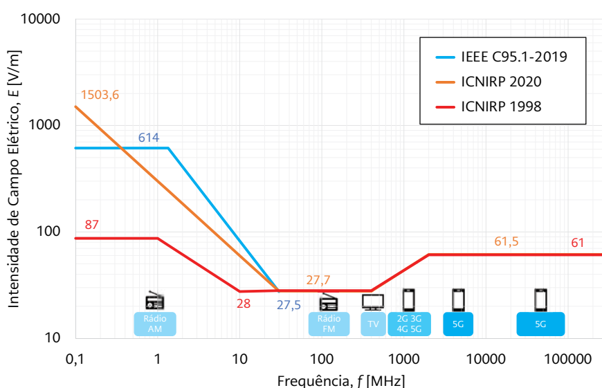
Figura 3 Níveis de intensidade de campo elétrico recomendados pelo ICNIRP e pelo IEEE-ICES para a exposição da população em geral.
