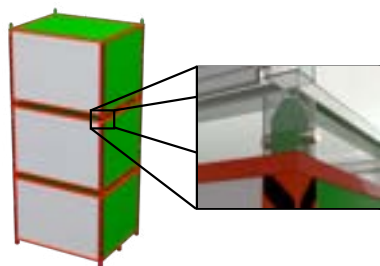
Figura 3: Empilhamento dos módulos de carga e detalhe do mecanismo de acoplamento.
