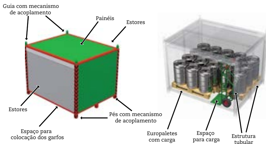
Figura 2: Módulo de carga: vista com os estores fechados (esquerda) e vista à transparência (direita).
