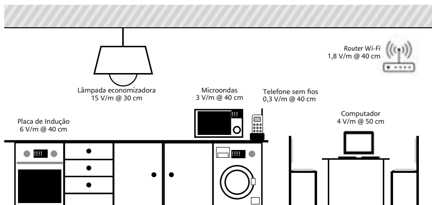
Figura 4 Intensidade de campo elétrico de alguns eletrodomésticos e equipamentos eletrônicos, adaptado de [8].
