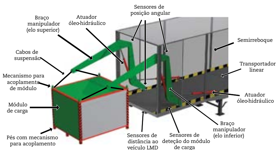
Figura 6: Braços manipuladores
