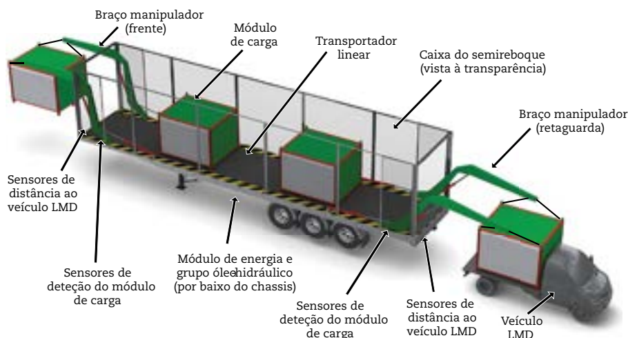
Figura 5: Sistema robótico de crossdocking
