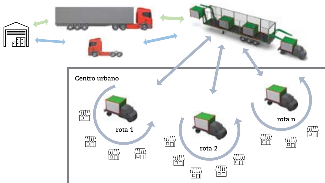
Figura 1: Conceito de distribuição com recurso a um sistema robótico para crossdocking móvel.
