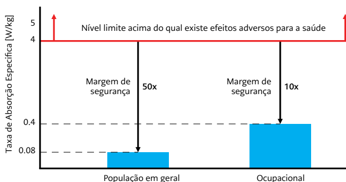
Figura 2 Níveis de referência da TAE recomendados pelo ICNIRP para exposição ocupacional e da população em geral.
