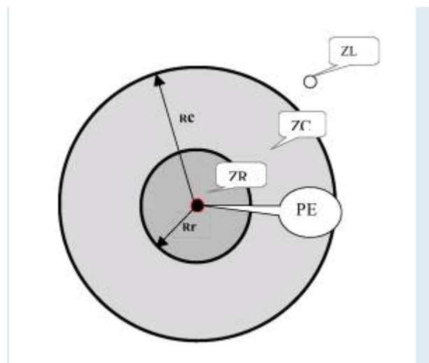
Figura 1 - Distâncias no ar que delimitam radialmente as zonas de risco, controlada e livre
